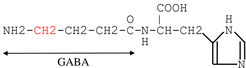
Homocarnosine
