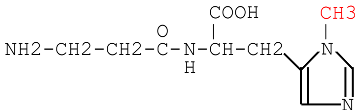
Anserine
