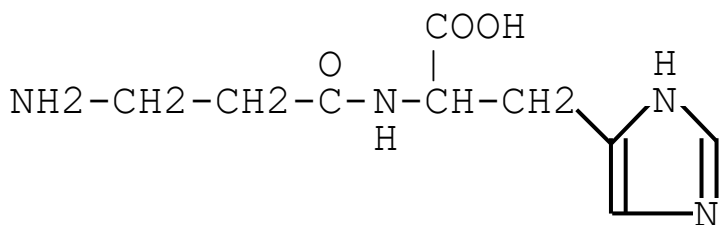
Carnosine
